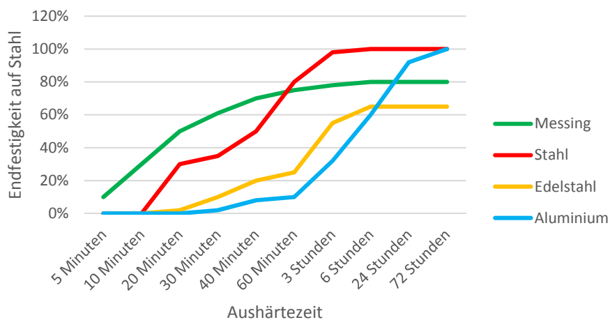
Aushärtegeschwindigkeiten/Schrauben M10
